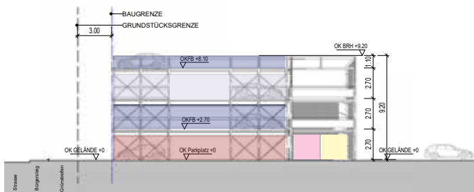
Ansicht Südosten
